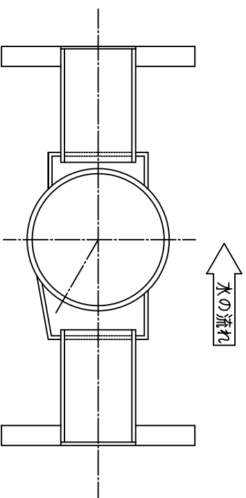
断面詳細 A-A
